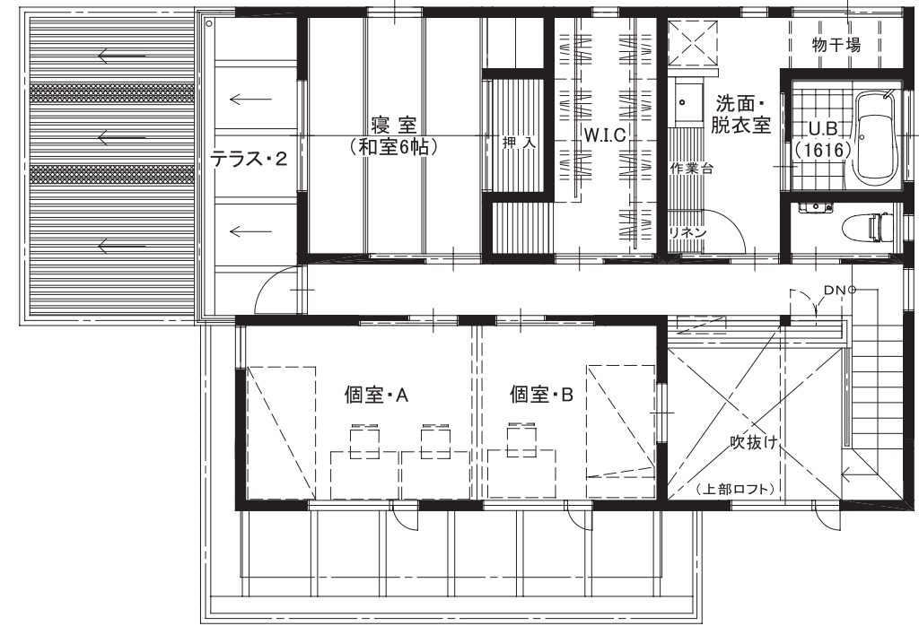
2階平面図
